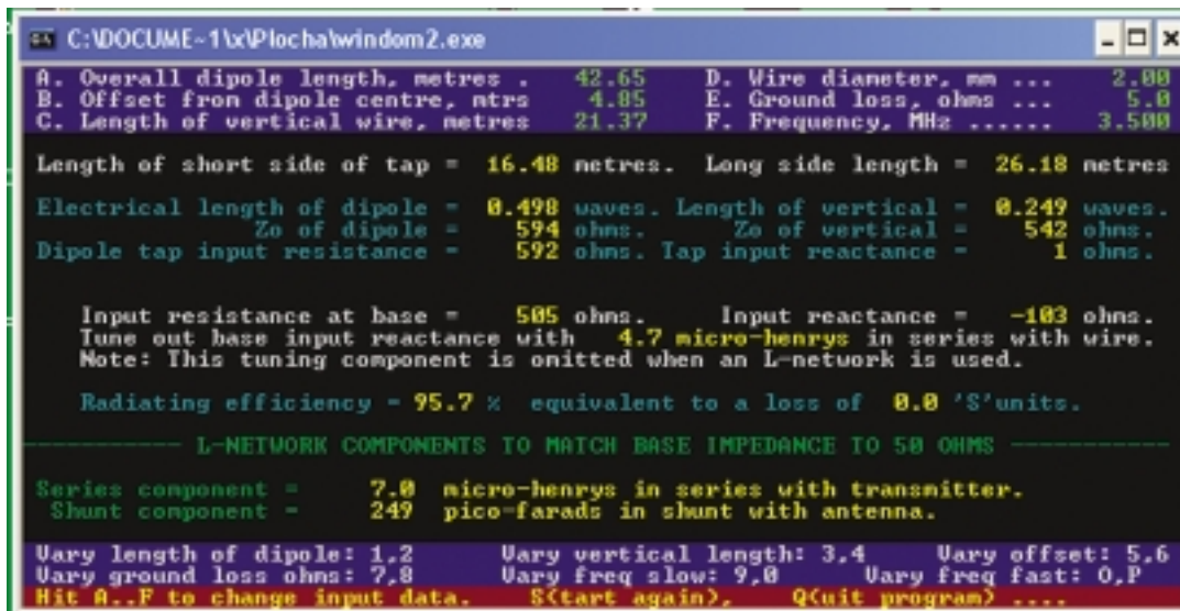
Obr. 3. Hlavní okno programu WINDOM 2 se všemi zadanými a vypočtenými údaji
