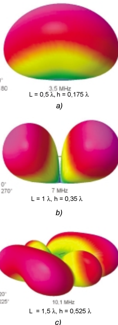
Obr. 2a až 2f. Prostorové (3D) diagramy záření této antény. Kromě kmitočtu je u každého diagramu uvedena délka (L) a výška (h) antény ve vlnové délce ( \lambda ), a dále elevace (el) a azimut (az) pohledu na prostorový diagram ve stupních
